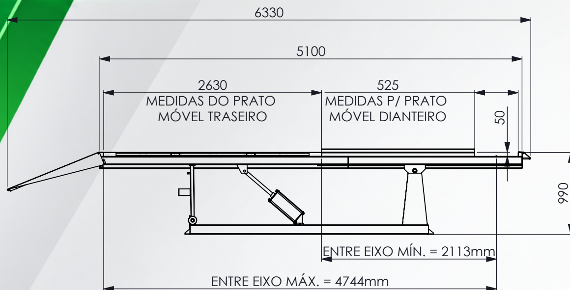
VISTA LATERAL POSIÇÃO AVANÇADO
