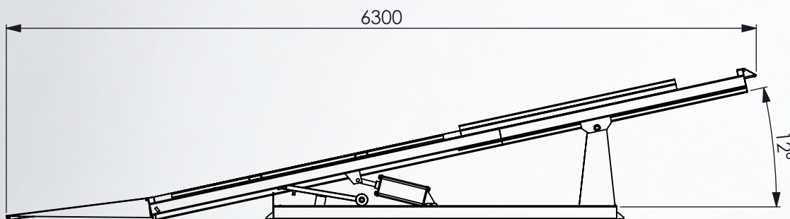
VISTA LATERAL POSIÇÃO RECUADO
